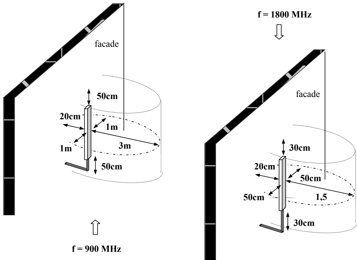
antenne panneau de macro cellule en façade
