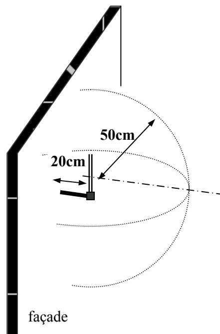
antenne fouet en façade
