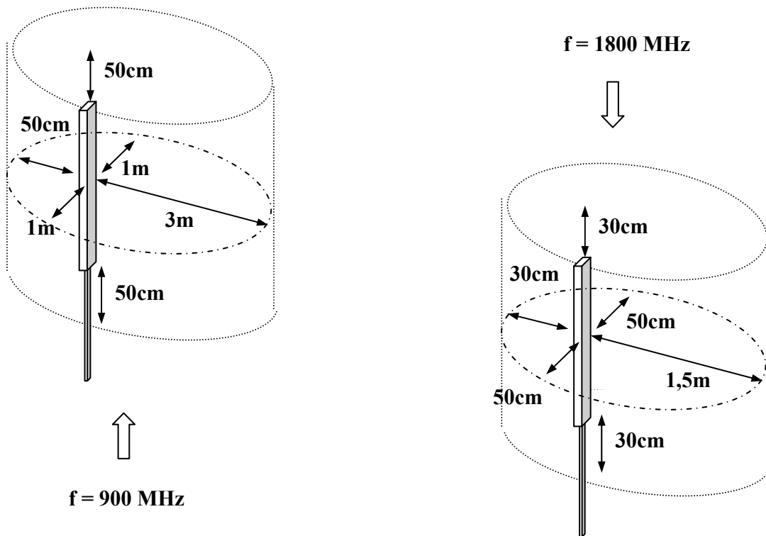
antenne panneau de macro cellule sur terrasse
